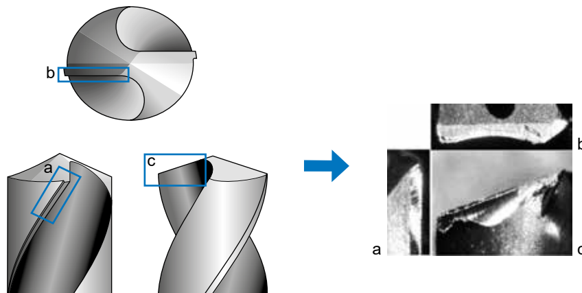
Schneidkantenbeschädigung
